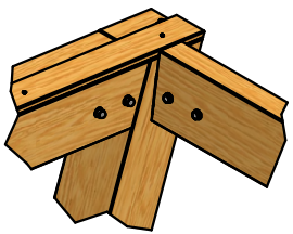
B (1 : 10)
