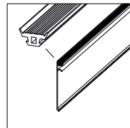
14. Afwerkkliklijst
