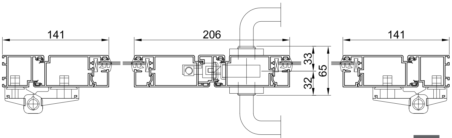
Detail 1 mit Flügelverbreiterung with leaf frame extension
