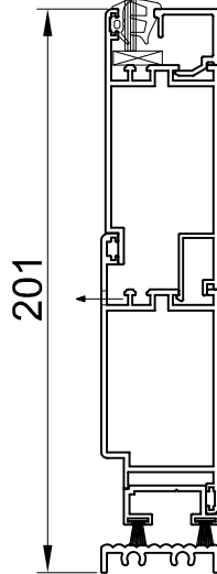
Detail 1 mit Flügelverbreiterung with leaf frame extension
